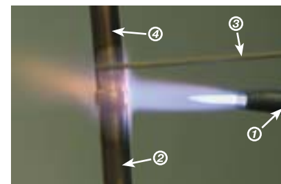
Расположение горелки и прутка припоя при пайке соединения концов труб, нагретых до тусклого вишнево-красного цвета: 1 – горелка; 2 – внутренняя труба; 3 – пруток припоя; 4 – наружная труба
